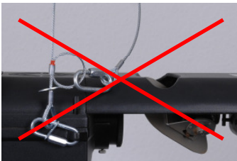
Bild 6: Schnellverbindungsglied nicht in Schlaufe einhaken.
