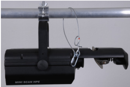
Bild 2: Zweisträngige Sicherungsmethode
